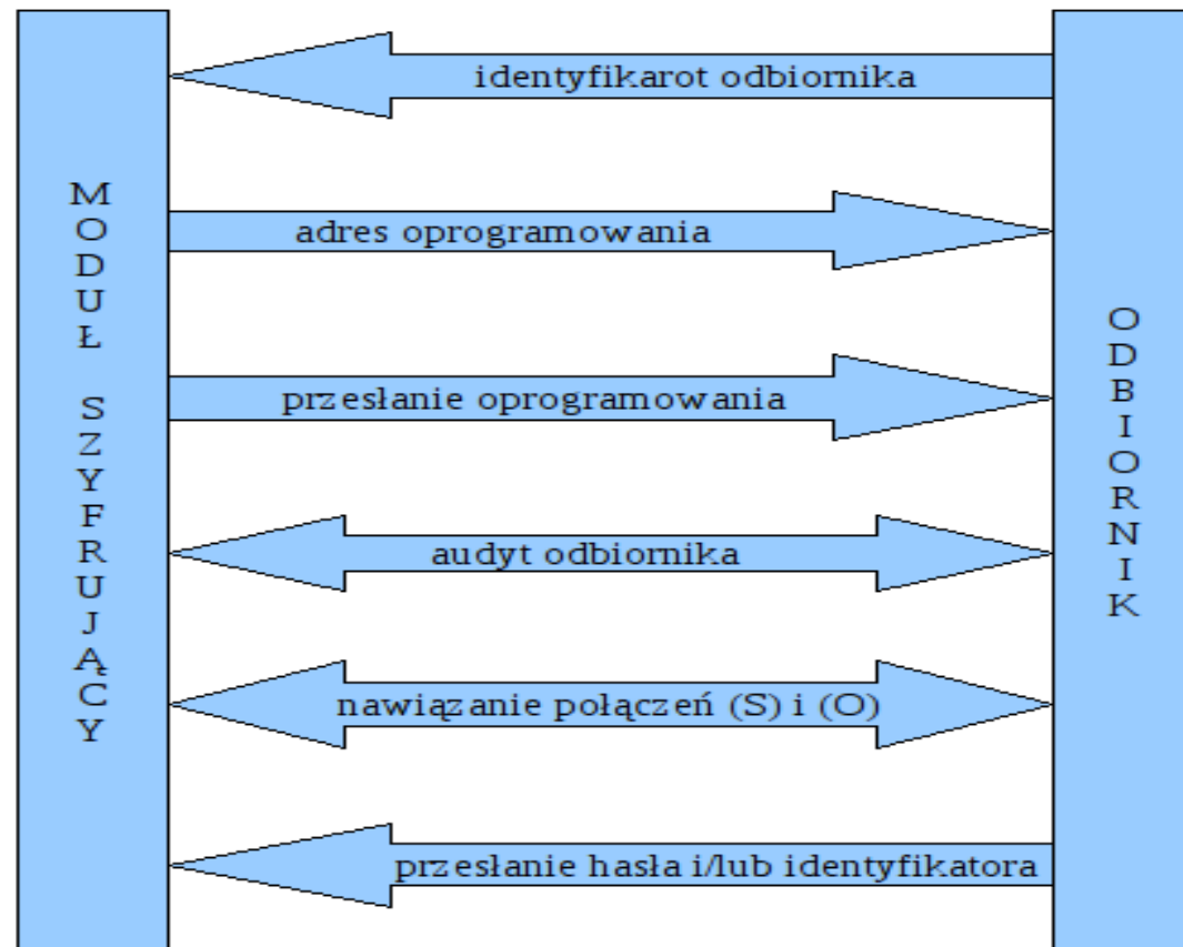
Schemat autoryzacji odbiornika (STB) w systemie KORSEC
